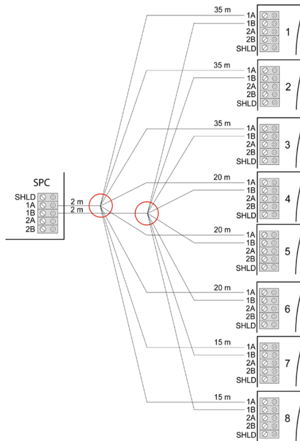
Sternverkabelung
