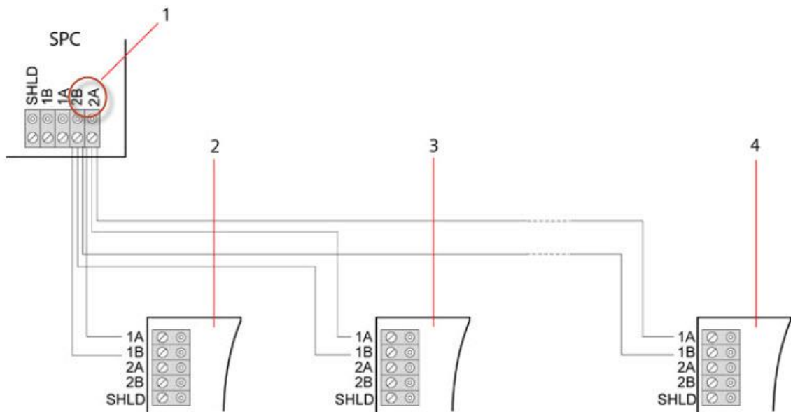
Sternkonfiguration 2
