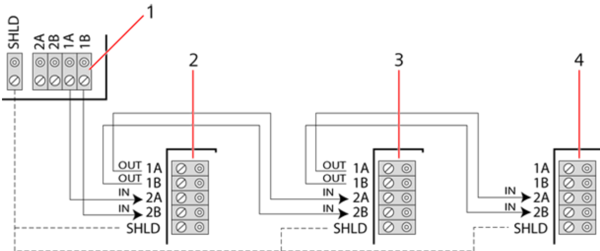
Stichleitungskonfiguration
